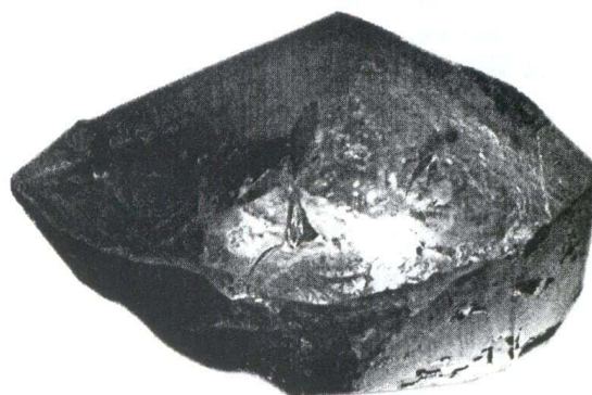
35. Кристал топаза. Центральний науково-природничий музей НАН України. Геологічний музей.
